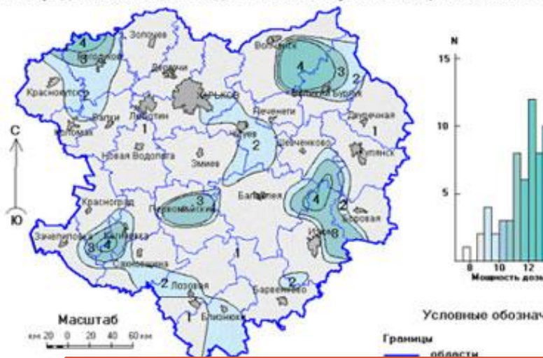
Распределение мощности дозы гамма-излучения в Харьковской области
