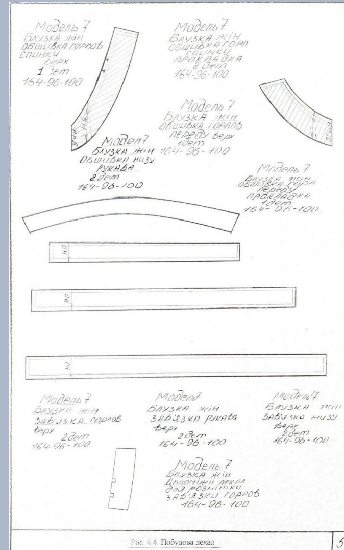
Рис. 4.4 Побудова лекал
